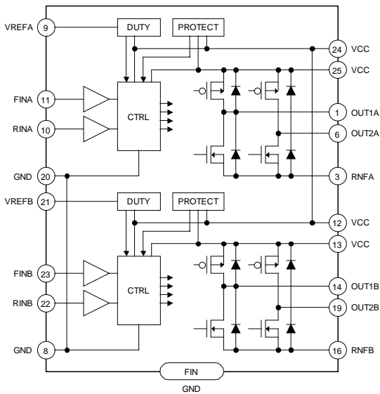
Fig. 33 BD6225FP, BD6226FP
