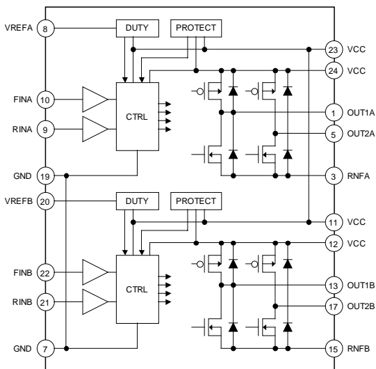
Fig. 31 BD6225FV
