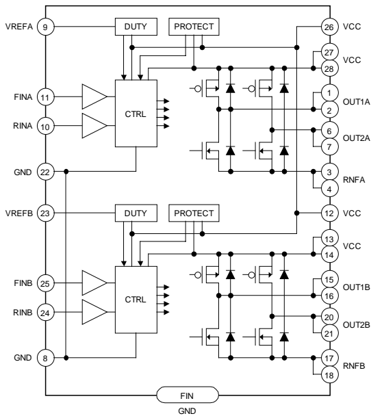
Fig. 36 BD6227FM
